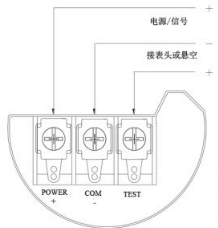
图 5-2 接线示意图
